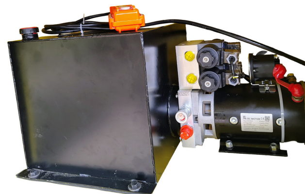
UNIDAD POTENCIA
