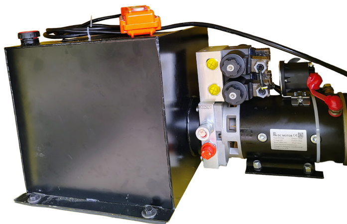
UNIDAD POTENCIA
