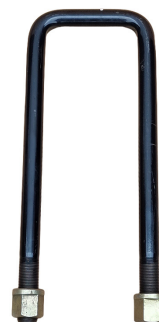
LAÑA DE 7/8 X 5 X 14"
